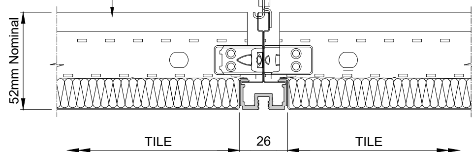
SECTION 'B' SCALE 1:2
