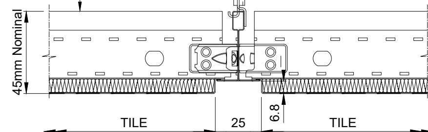
SECTION 'B' SCALE 1:2
