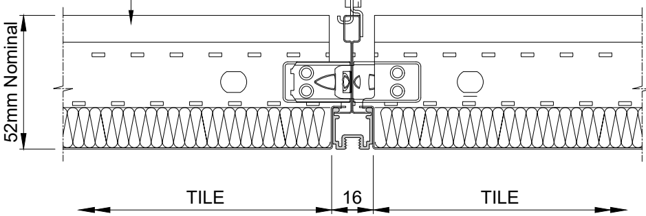
SECTION 'B' SCALE 1:2
