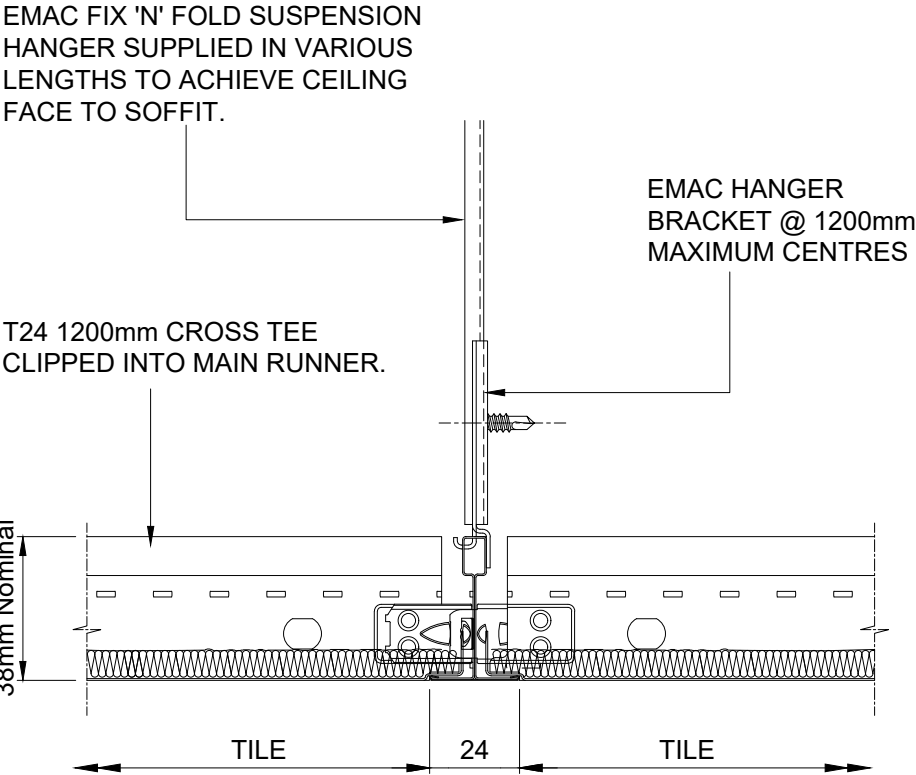
SECTION 'B' SCALE 1:2
