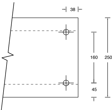
CEE 250
