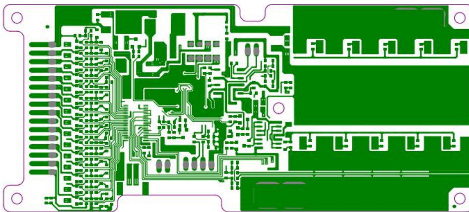
顶层走线图
