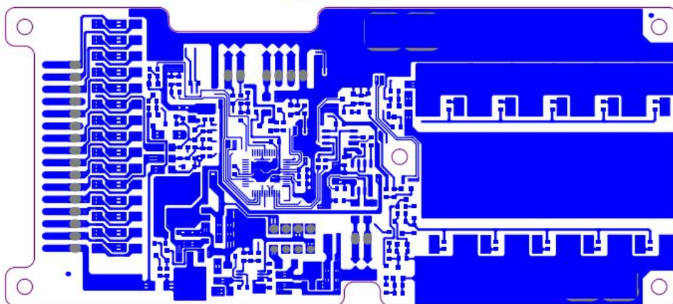
底层走线图
