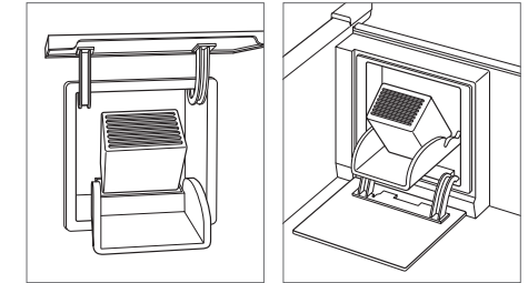
Luchtzuiveringscartridge (zuil en hoog).
