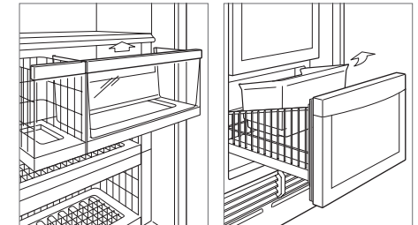
Contenitore a colonna del ghiaccio.
