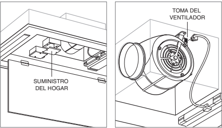
Conexiones eléctricas
