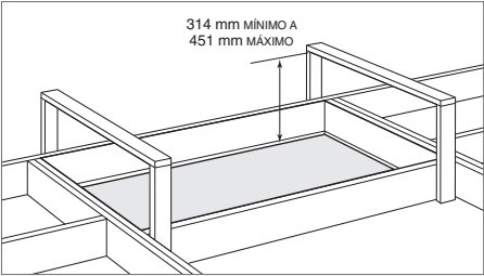
Marco de soporte (típico)
