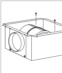
Installatie interne ventilator
