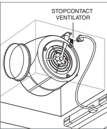
Aansluiting ventilator
