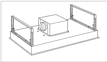
Installation der Halterungen
