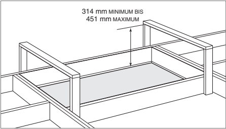
Stützrahmenwerk (typisch)
