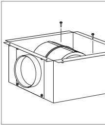
内置式鼓风机安装
