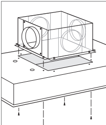
Richting van afvoer
