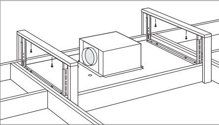
通风罩安装
