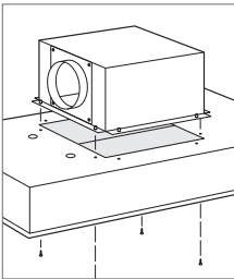
Verwijdering ventilatordoos
