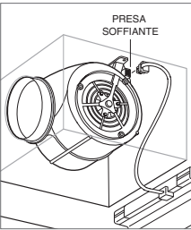
Connessione della soffiante
