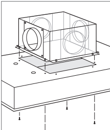
Dirección de la descarga interna
