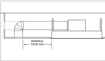
Recirculatietoepassing
