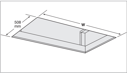
Dimensioni vano incasso
