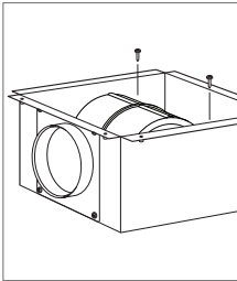
Installazione della soffiante interna
