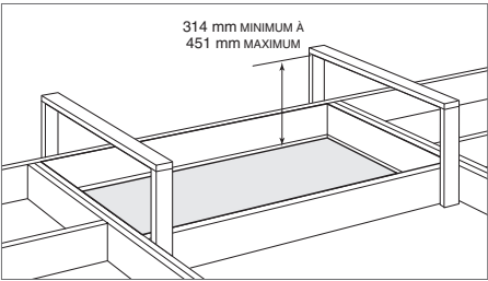
Support structurel (typique)
