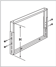
支架调整
